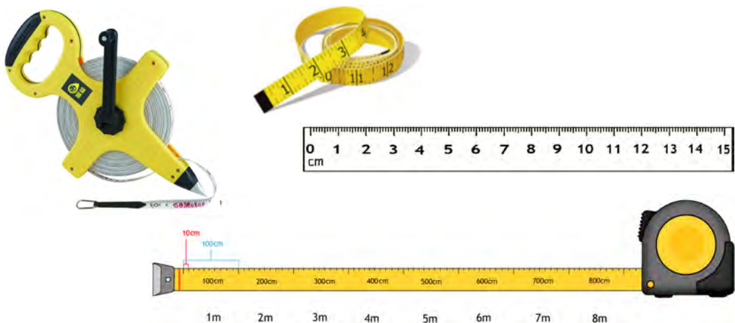
चित्र न. 1.7 लम्बाइ नाप्न प्रयोग गरिने उपकरणहरू
