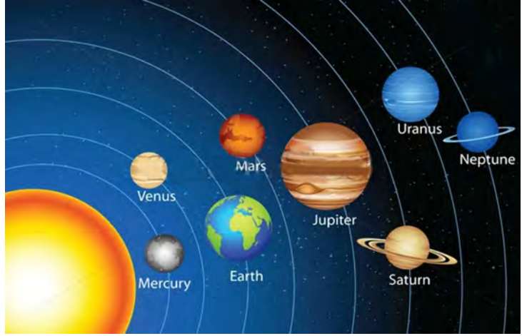
चित्र 11.11 सौर्य मण्डल
